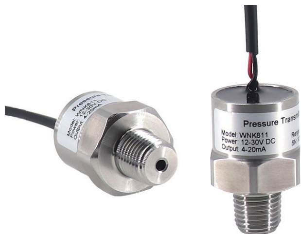
WVK811-B 范围：-100KPa~60MPa 精度：0.5% 扩散硅型
